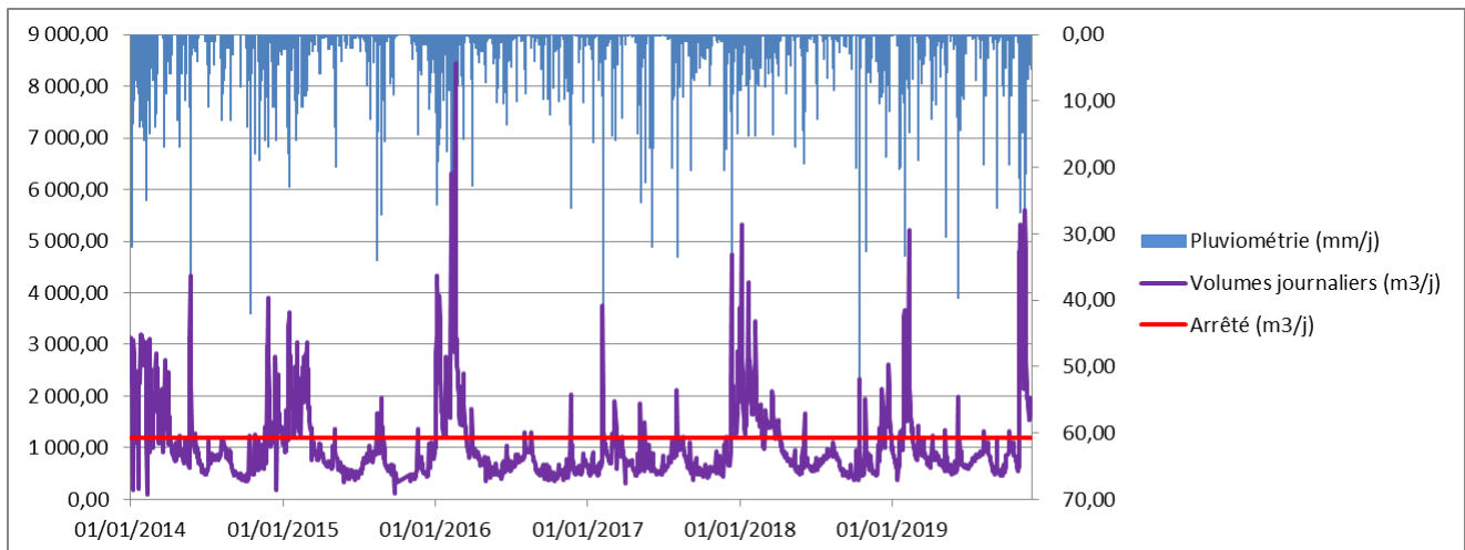
Figure 8 : Débits mesurés en entrée de la STEP de Trébeurden (source : LTC)
