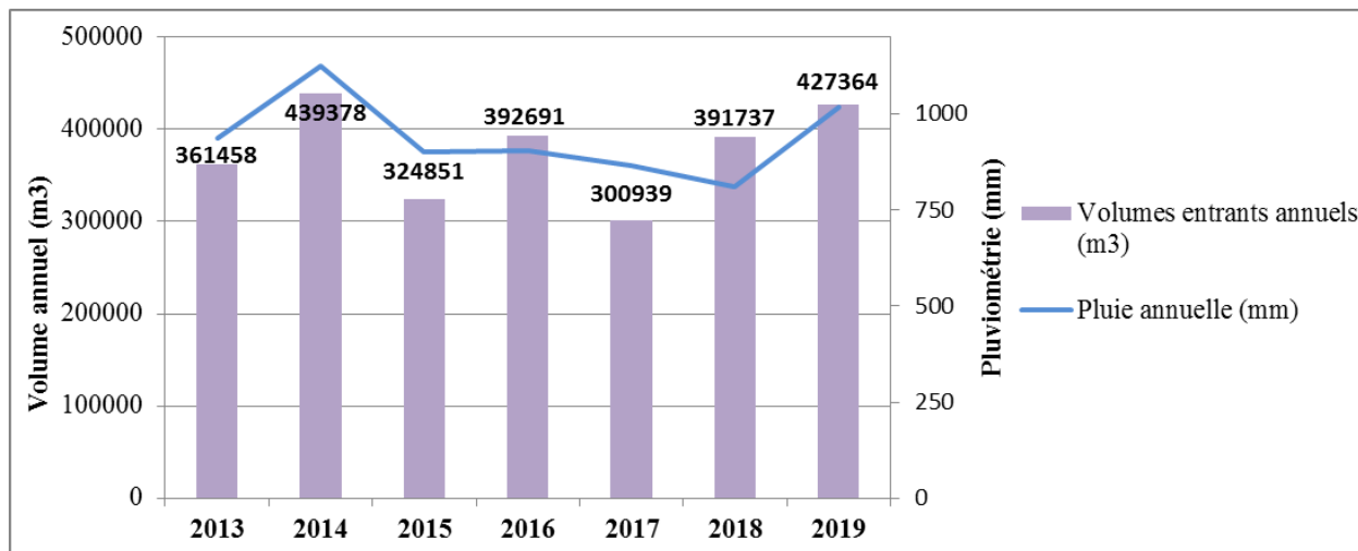
Figure 7 : Volumes annuels en entrée de station entre 2013 et 2019 (source : LTC)
