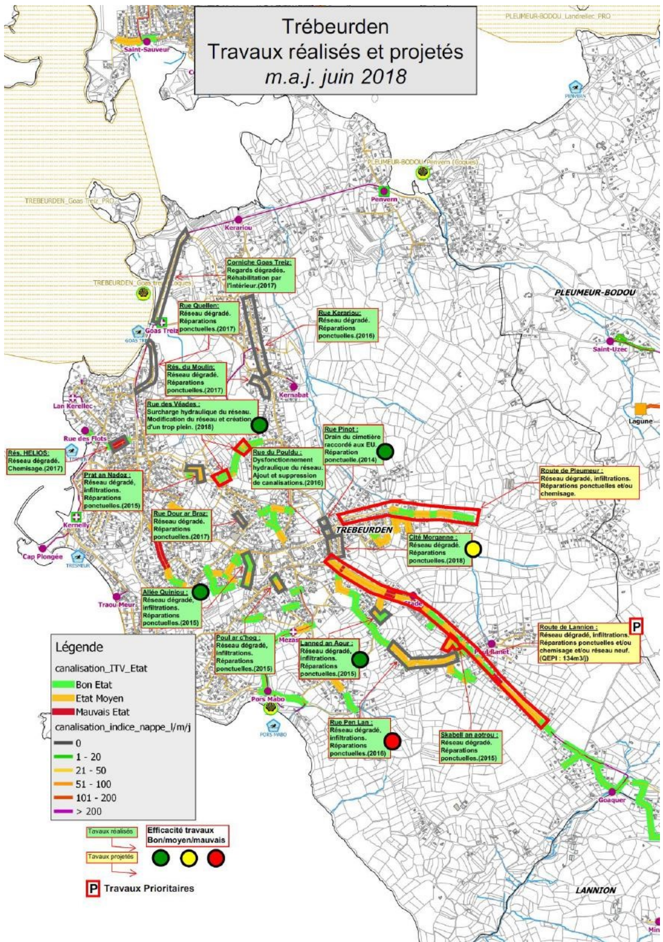
Figure 9 : Travaux projetés et réalisés sur le système d'assainissement de Trébeurden
