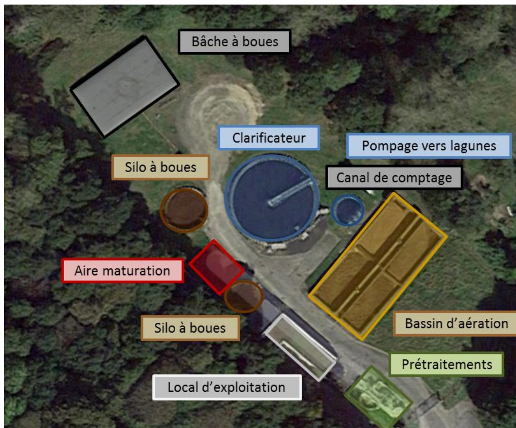
Figure 13 : Localisation des différents ouvrages de la station
