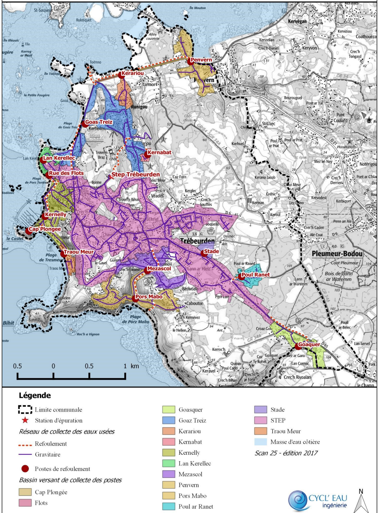
Figure 6 : Présentation des bassins de collecte par poste de relèvement à Trébeurden
