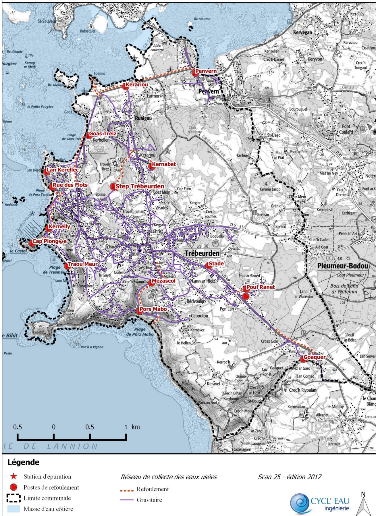
Figure 5 : Présentation du réseau de collecte et des postes de refoulement du système d'assainissement de Trébeurden
